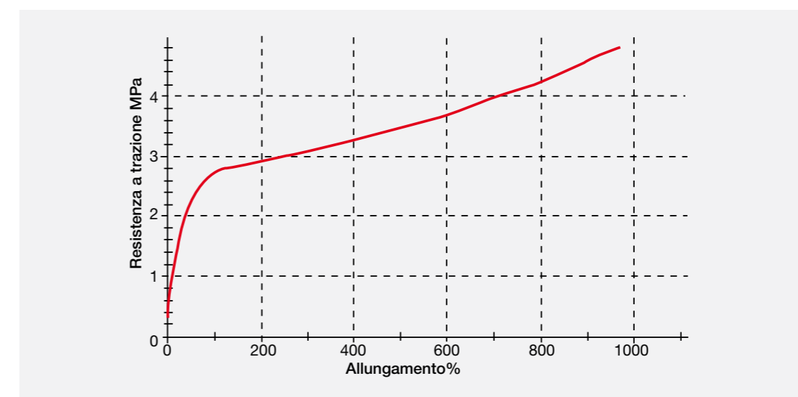
Diagramma sforzo deformazione a trazione della membrana
